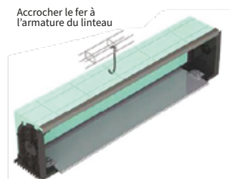
Alignement nu extérieur
