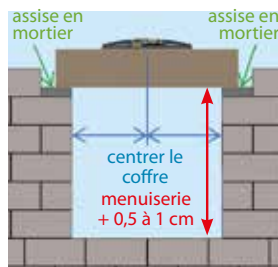
Centrage du coffre
