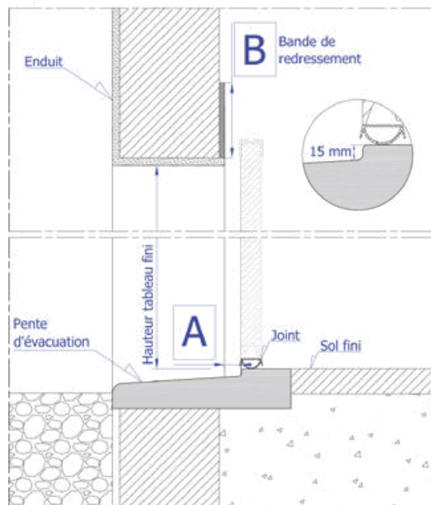
Coupe verticale
