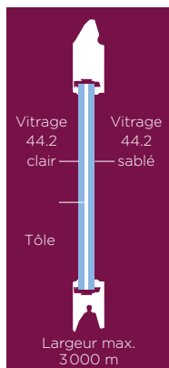
Vitrage + tôle
