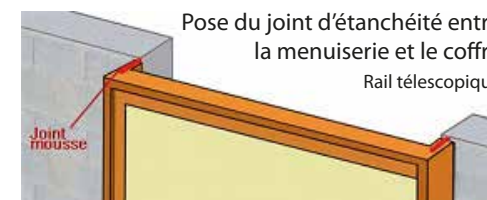
Pose d'étanchéité sur la menuiserie
