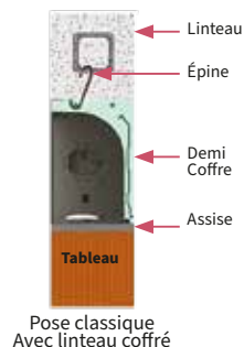
Centrage du coffre
