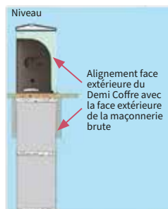
Alignement nu extérieur
