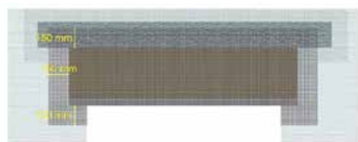
Renforcement de l'enduit jusqu'à 2500 mm
