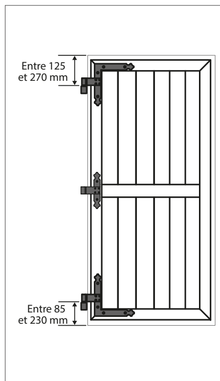
EQUERRE DE 300 MM
