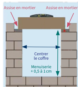
Centrage du coffre
