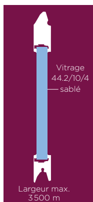
Double vitrage
