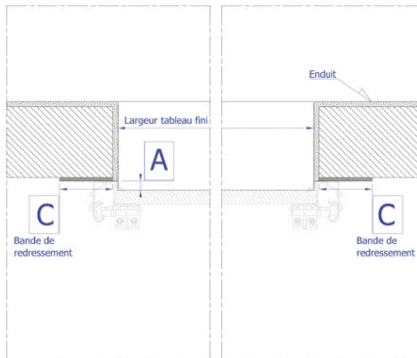
Coupe horizontale
