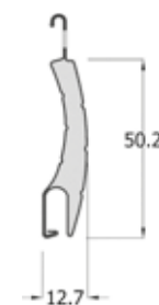
Coupe de la lame
